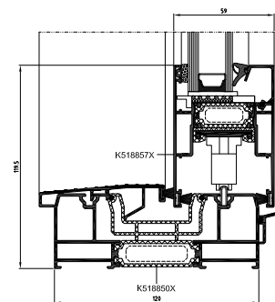
przekrój dolny drzwi
