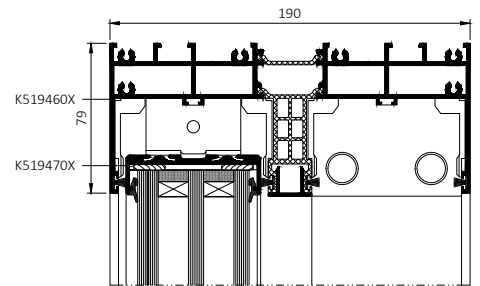
przekrój górny drzwi
