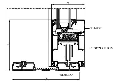
przekrój dolny drzwi z niskim progim
