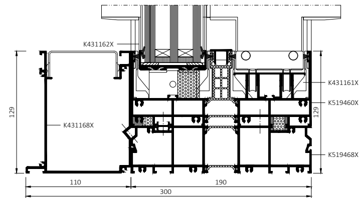
przekrój dolny drzwi
