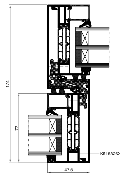
przekrój przez połączenie skrzydeł
