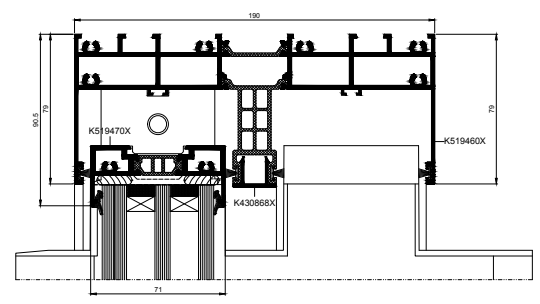
przekrój górny drzwi
