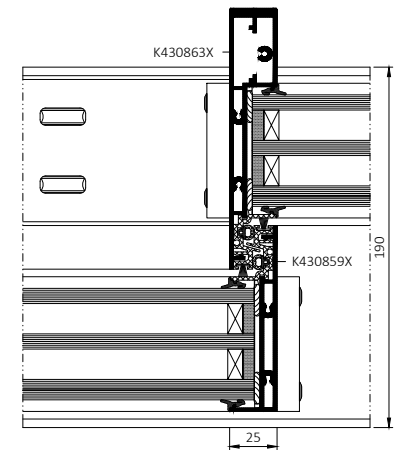
przekrój przez połączenie skrzydeł drzwi
